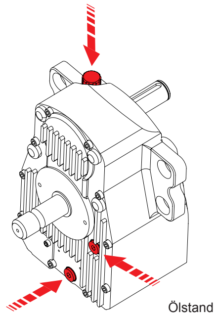
Ablassschraube
