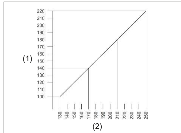
(1) Pression de sortie de la graisse, en bar / (2) Pression d'entrée de l'hydraulique, en bar.
