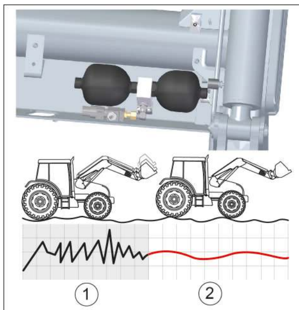
(1) Sans SHOCK ELIMINATOR System / (2) Avec SHOCK ELIMINATOR System
